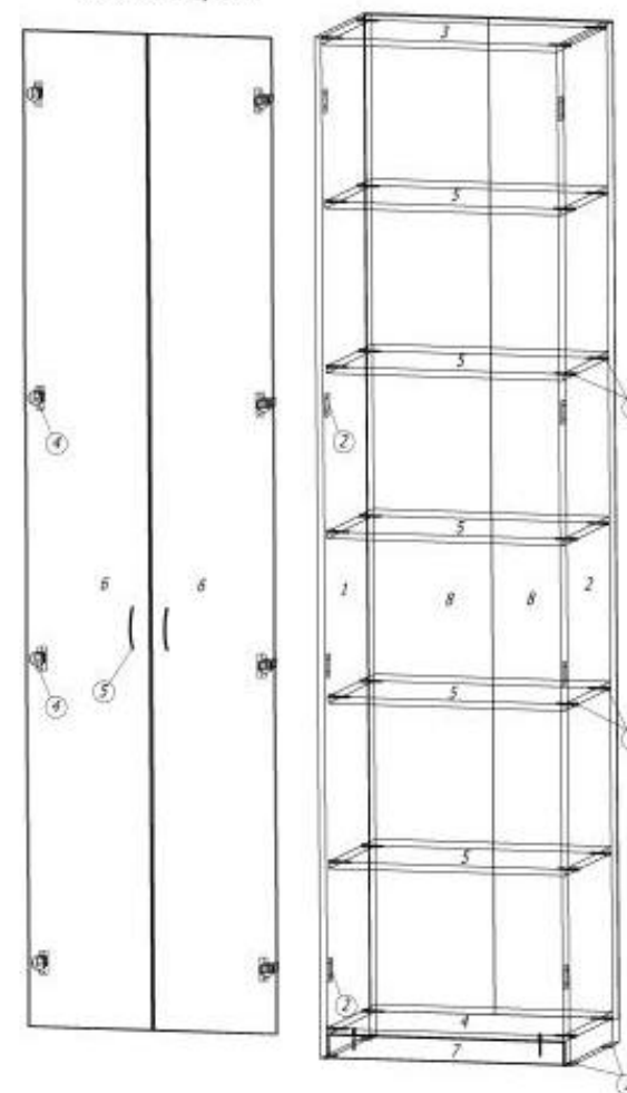
Схема сборки
